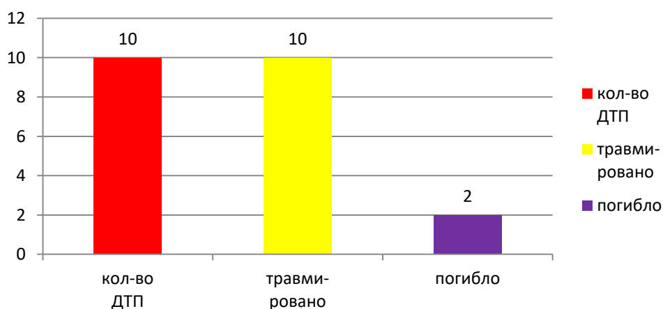
Диаграмма 4. ДТП в аналогичный период 2021 года
