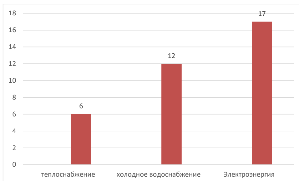
Диаграмма 3. Происшествия на объектах ТЭК и ЖКХ.
