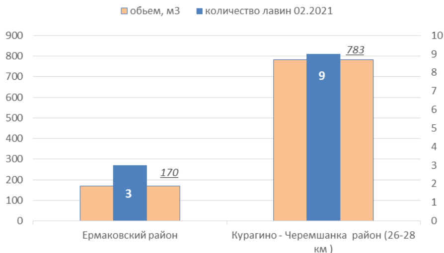
Диаграмма 2. Сход снежных масс за аналогичный период 2021 года
